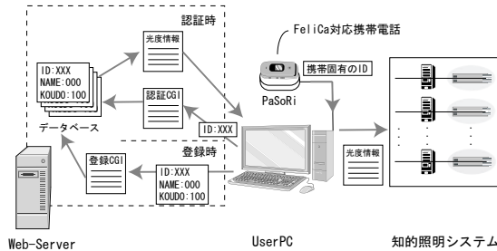
図 3: FeliCa による照明制御システム構成 (出典: 自作)
